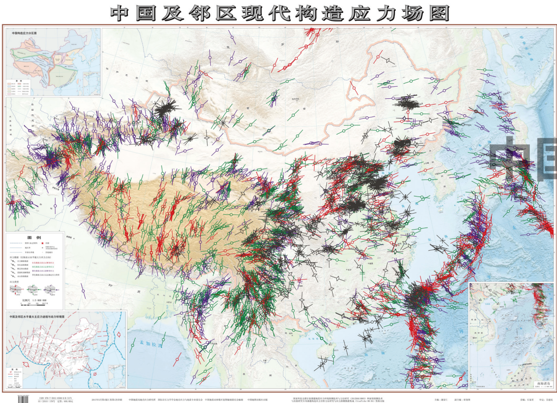
图18 中国及邻区现代构造应力场图
