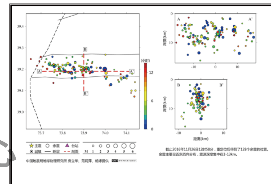
图21 余震精定位图
