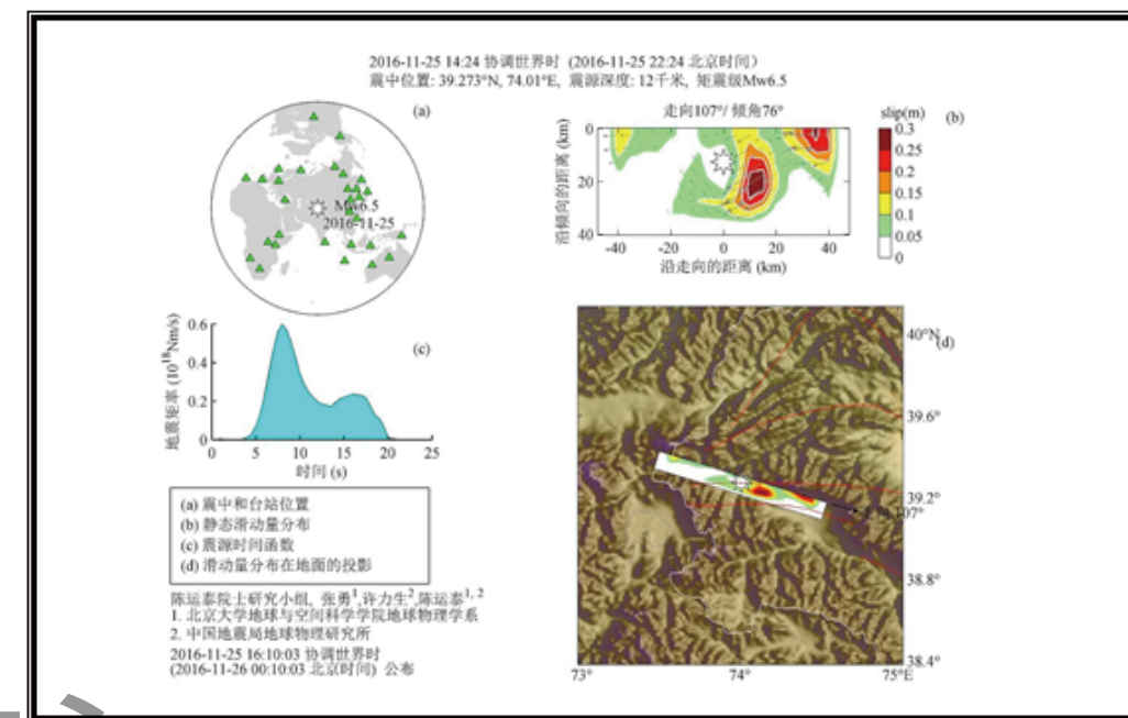
图24 震源破裂过程图
