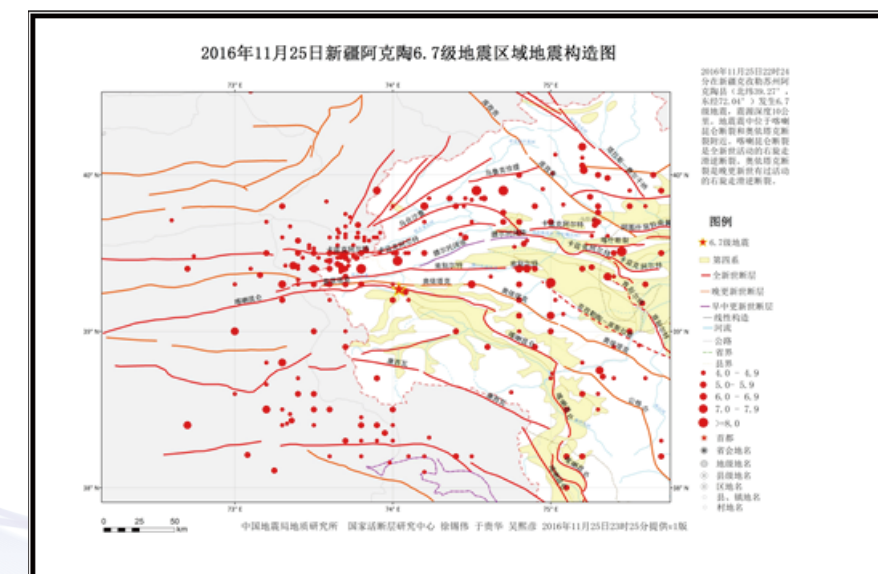
图22 区域地震构造图
