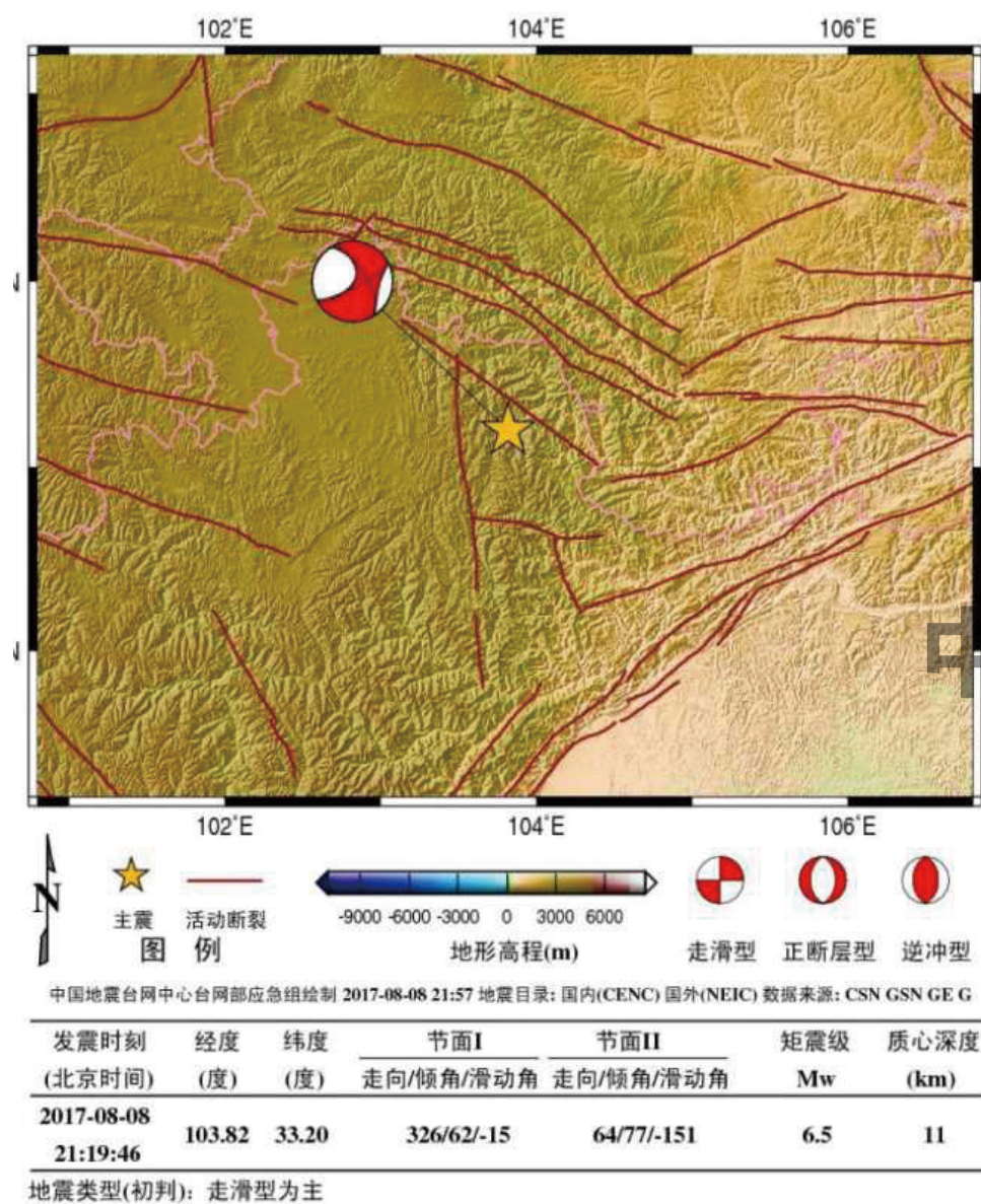
图23 主震震源机制解图
