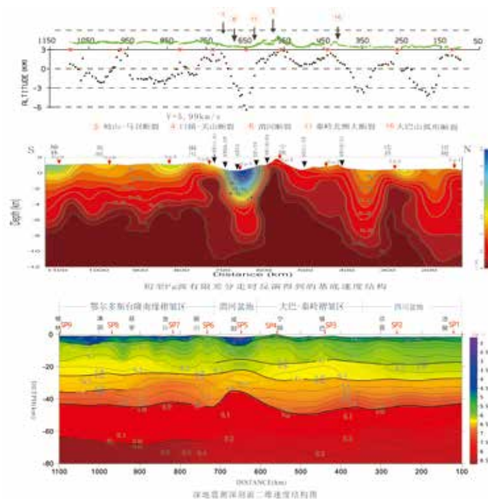
图18 探测剖面二维速度结构图
