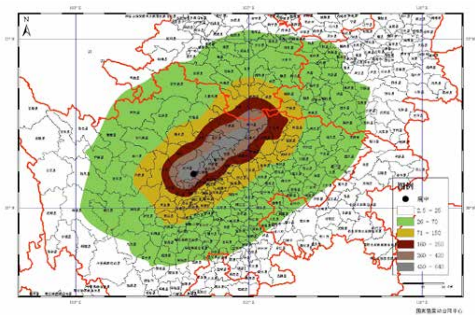
图8 汶川8.0级地震主震PGA(东西)分布图
